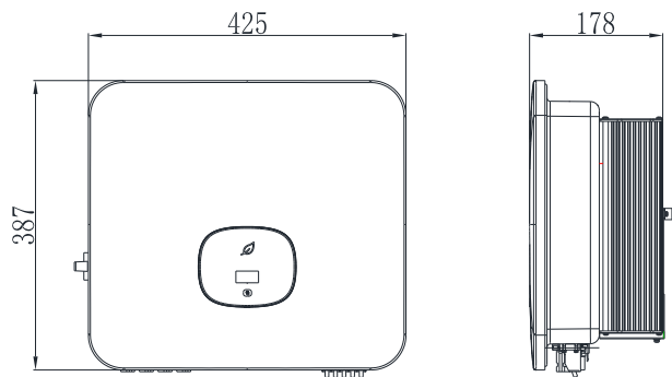
图 2.2 尺寸规格
