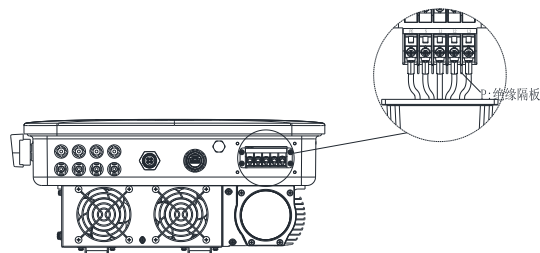
图 5.3 AC端子接线示意
