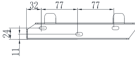
图 4.6 壁挂架规格图
