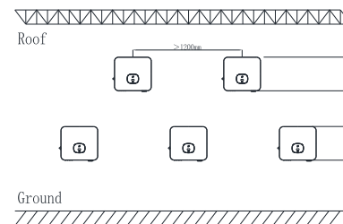
图 4.3 多台逆变器时的安装尺寸
