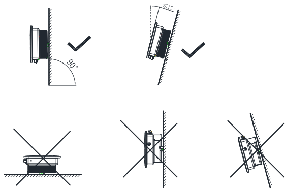
图 4.1 安装示意图
