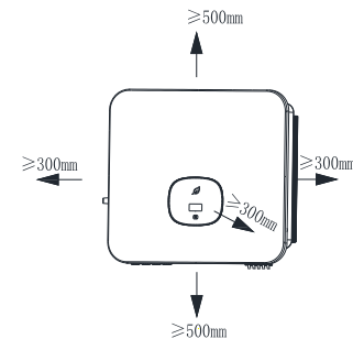
图 4.2 一台逆变器时安装尺寸
