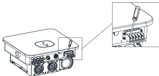
图5.4 AC端子接线示意二
