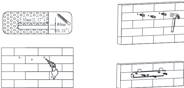
图 4.7 壁挂架安装示意图
