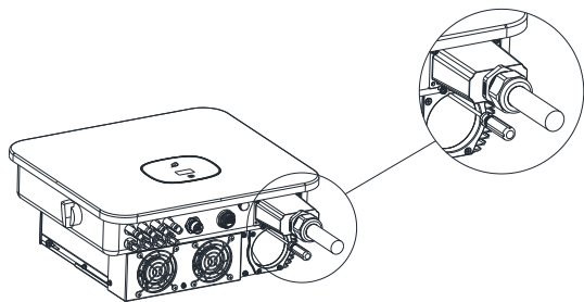
图5.5 AC端子接线示意三
