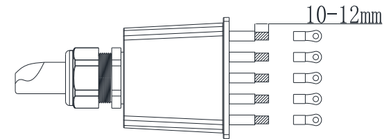
图 5.2 AC输出线压接端子示意
